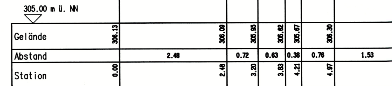
Profil 6 M. 1:50
