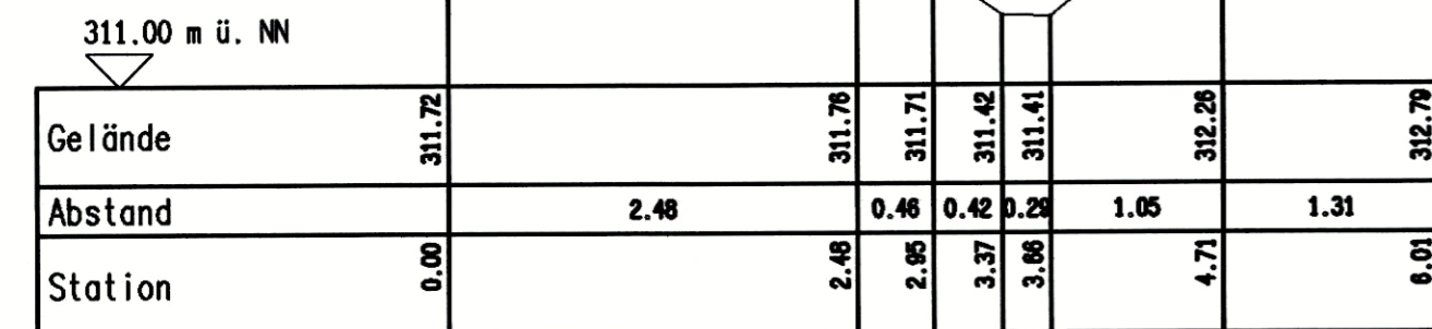
Profil 3 M. 1:50
