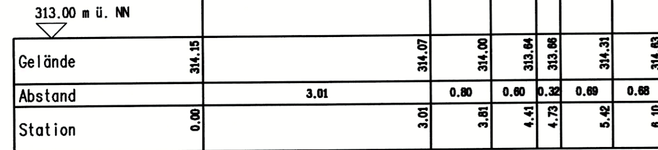
Profil 1 M. 1:50
