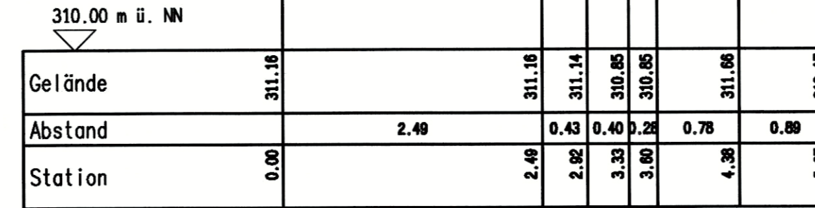
Profil 4 M. 1:50
