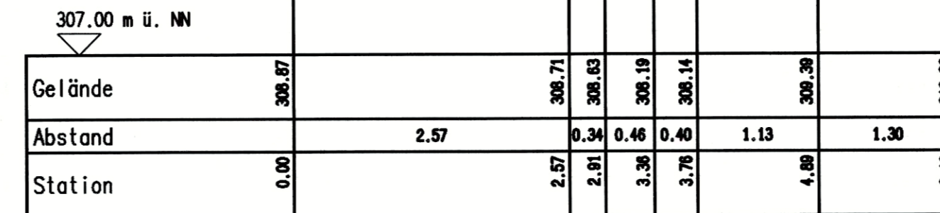
Profil 5 M. 1:50
